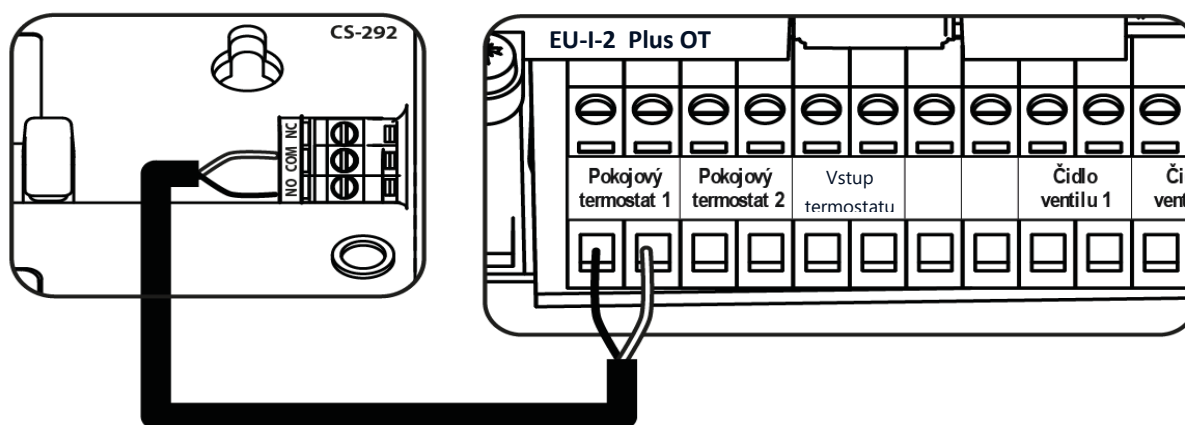
Příklad zapojení dvoupolohového (ON/OFF) termostatu
